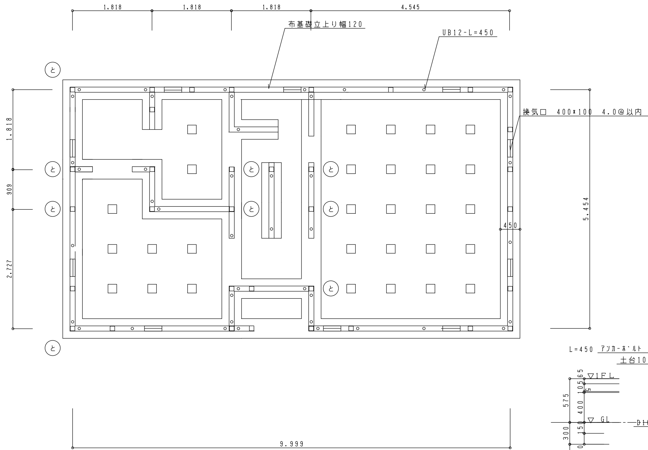
基礎 伏図 1/50
